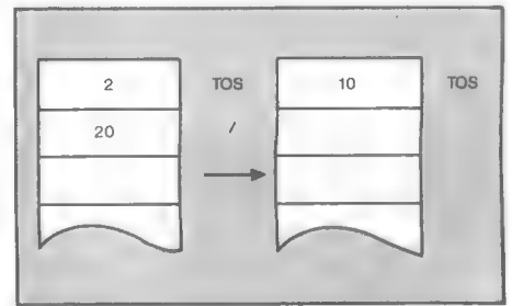
Bild 3. So verändert sich der Stack bei der Division
